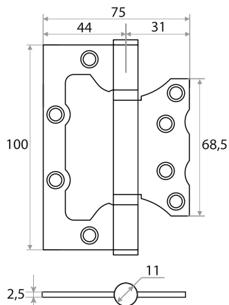
ПЕТЛЯ НАКЛАДНАЯ 100X75X2,5 БЕЗ ВРЕЗКИ, Б/К
