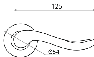
РУЧКА РАЗДЕЛЬНАЯ "61" СЕРИЯ 10
