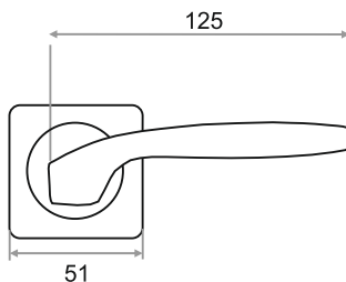
РУЧКА РАЗДЕЛЬНАЯ "228" СЕРИЯ 03 SLIM
