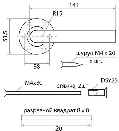
РУЧКА РАЗДЕЛЬНАЯ SS-1903 НЕРЖАВЕЮЩАЯ СТАЛЬ
