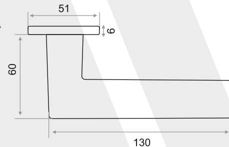
Ручка раздельная "2118 AL" серия 06 slim
